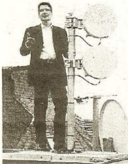
Bild: Oliver Fabry demonstriert die beiden Richtfunkantennen, die auf die Relaisstationen auf dem Hochhaus der Fachhochschule Frankfurt ausgerichtet sind und je eine indirekte 36+2 Mobil-Verbindung zu den Krankenhäusern Marius und Diakonissen realisieren (Foto improve)
